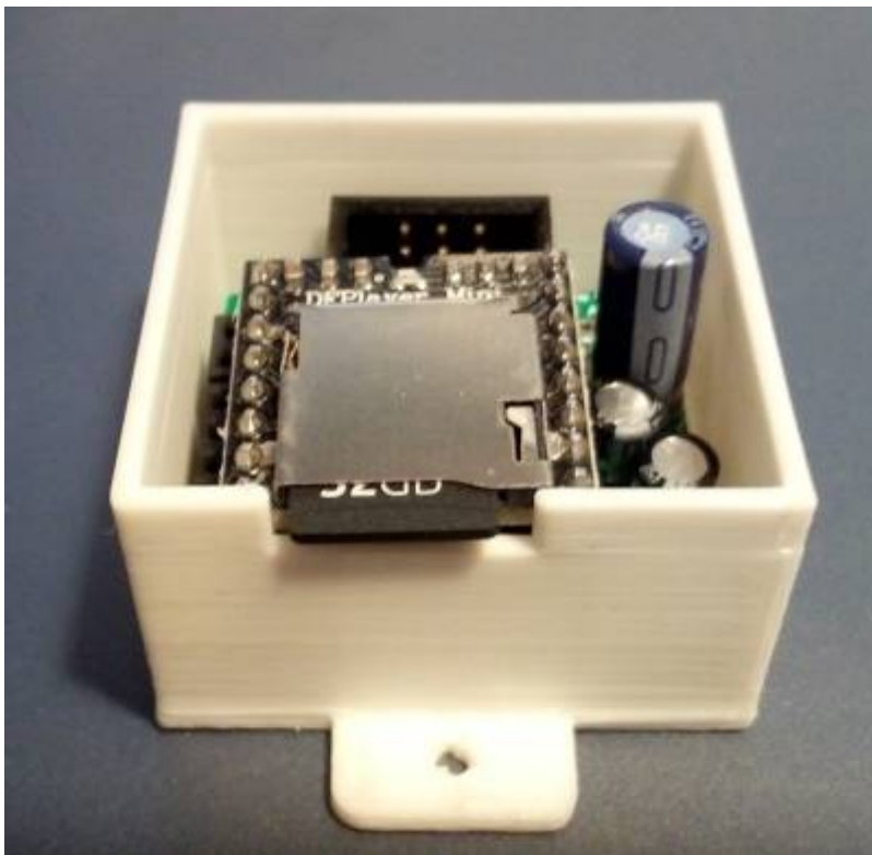
Gehäuse 501 - Wannenstecker
