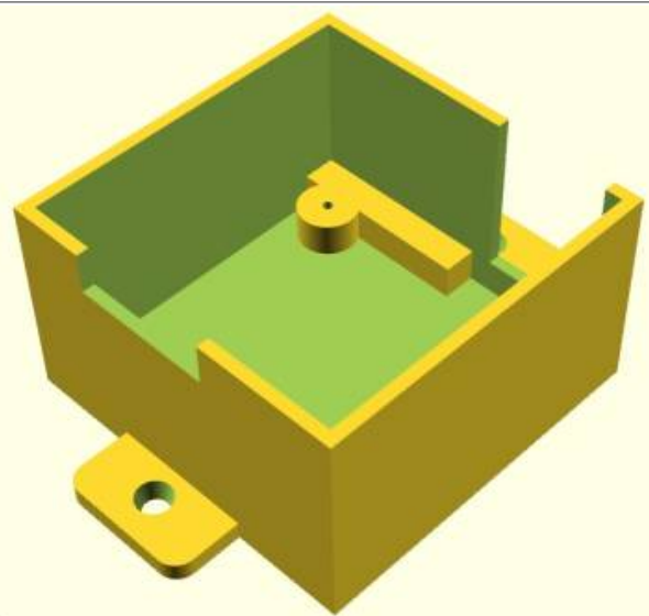
Gehäuse 501 - Westernbuchse
