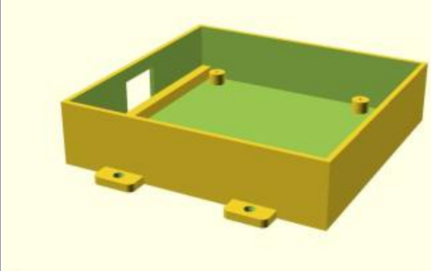
Gehäuse mit Öffnung für die Relaiskontakte der ABC-Bremse
