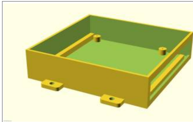
Gehäuse mit Öffnung für die 6 Relaiskontakte OUT_A - OUT_F
