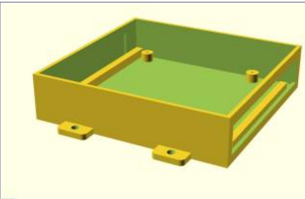
Gehäuse mit Öffnung für die 6 Relaiskontakte OUT_A - OUT_F und vorgestanzter Öffnung für OUT_G & OUT_H
