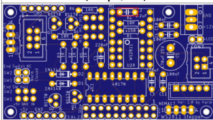
C2 (2.20μF / 225)
