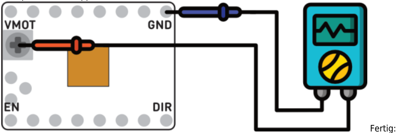
Messpunkte am Steppertreiber TMC2208:
