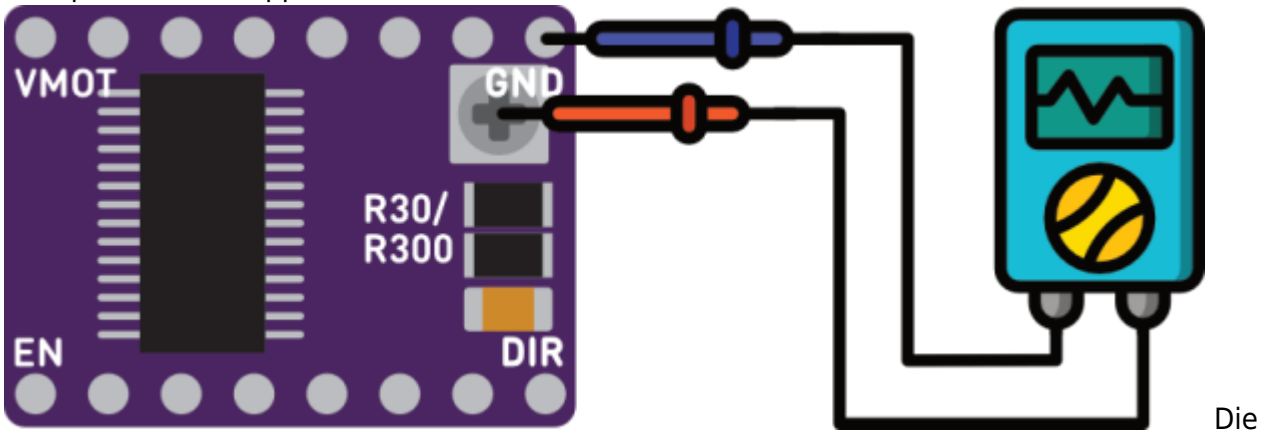
Messpunkte am Steppertreiber TMC2208:
