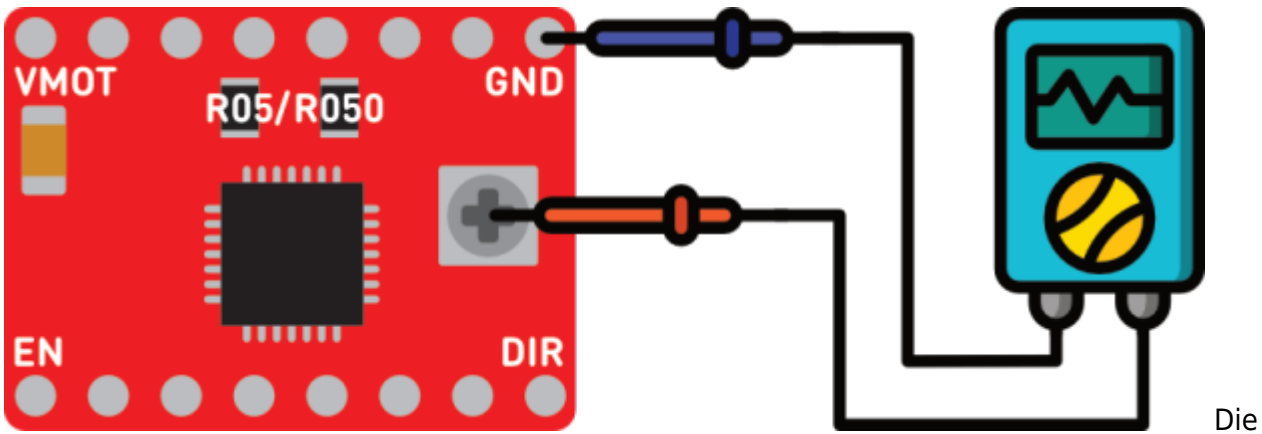
Messpunkte am Steppertreiber DRV882:
