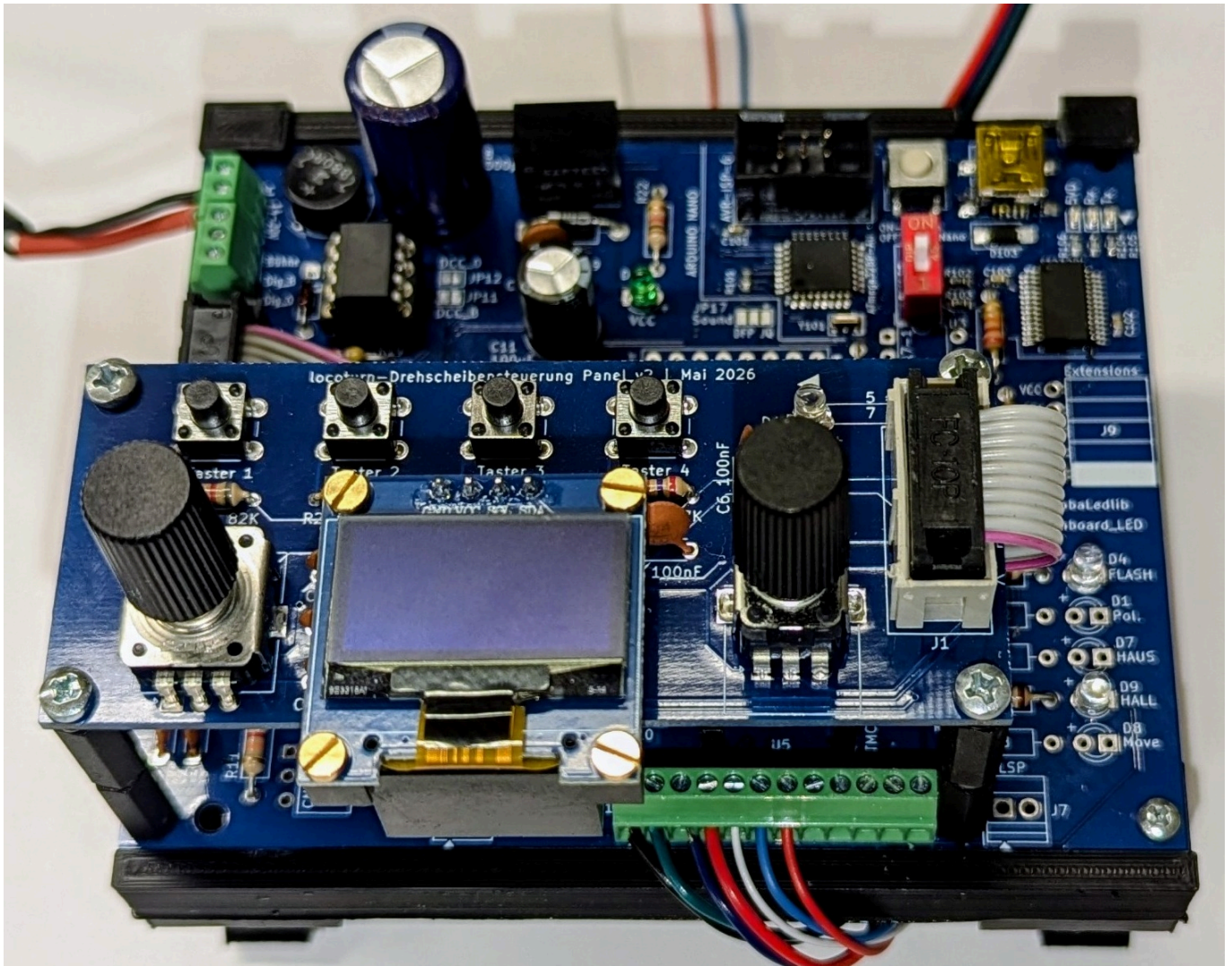
locoturn V2: Panel „huckepack“ und OLED mit 3D-gedruckter Halterung. Die abgebildete OLED-Halterung als stl-Datei zum Selberdrucken:
