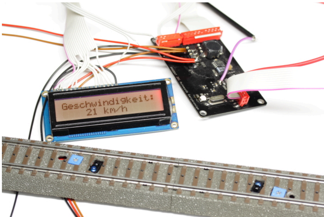
Die Finale Version mit Atmega328PB
